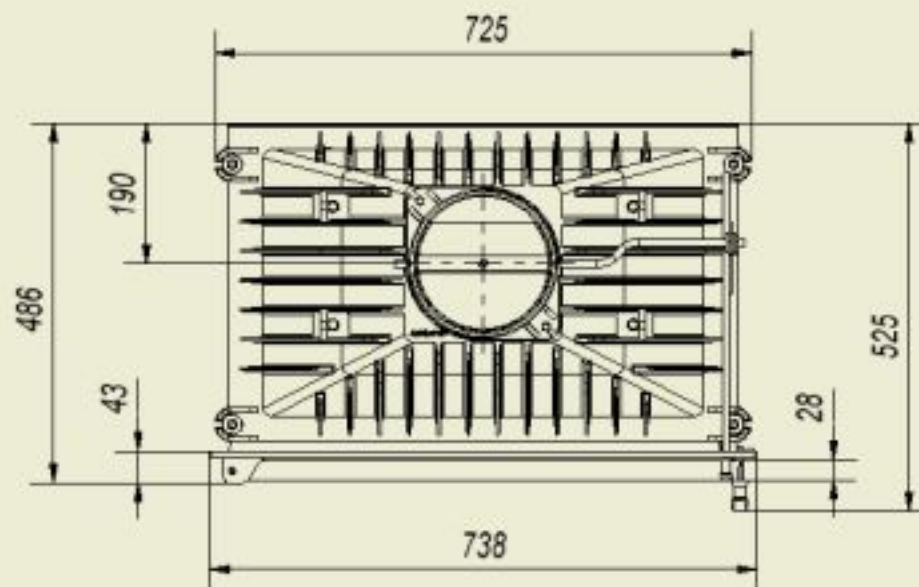
Wkład kominkowy OLIWIA 18 KW
