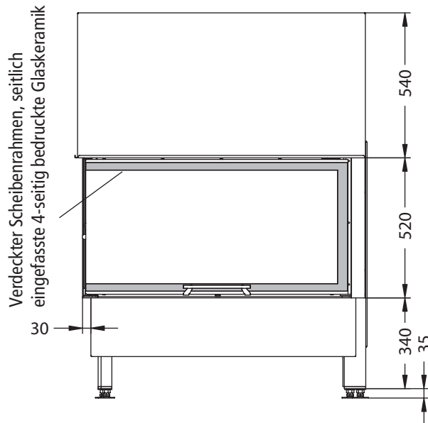
Vorderansicht M~1:20
