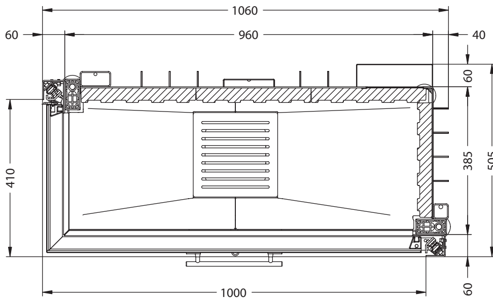
Horizontalschnitt M~1:10
