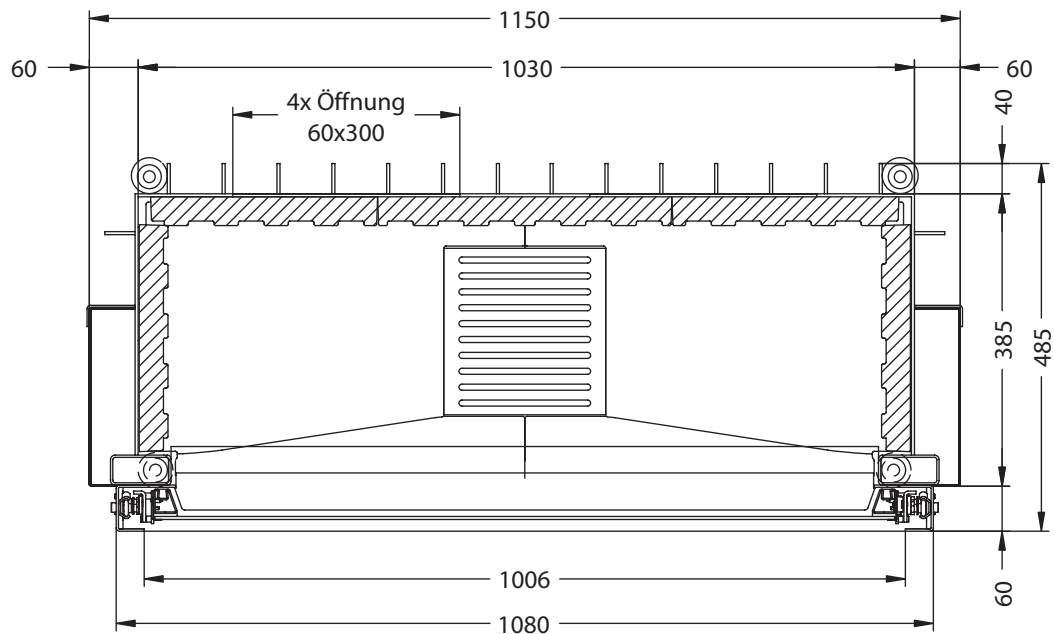
Horizontalschnitt M~1:10
